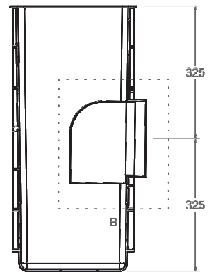
CORTE A-A
