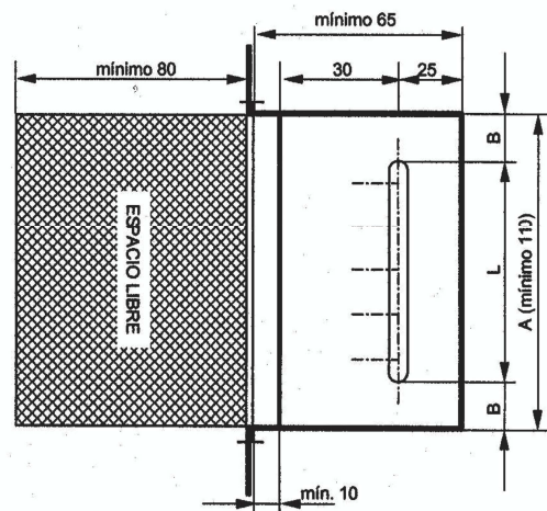
ARMARIO BATERÍA PLANTA
