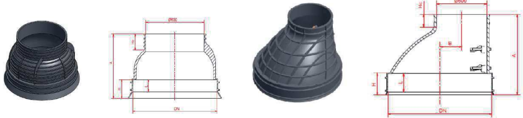
Cono reductor de pozo de diámetro 1000 y 1200 mm
