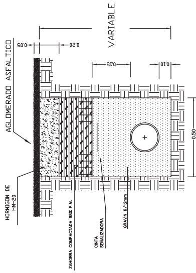
ZANJA TIPO SANEAM./PLUVIALES CON REPOSICIÓN
