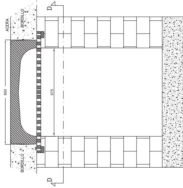
SECCION B-B
