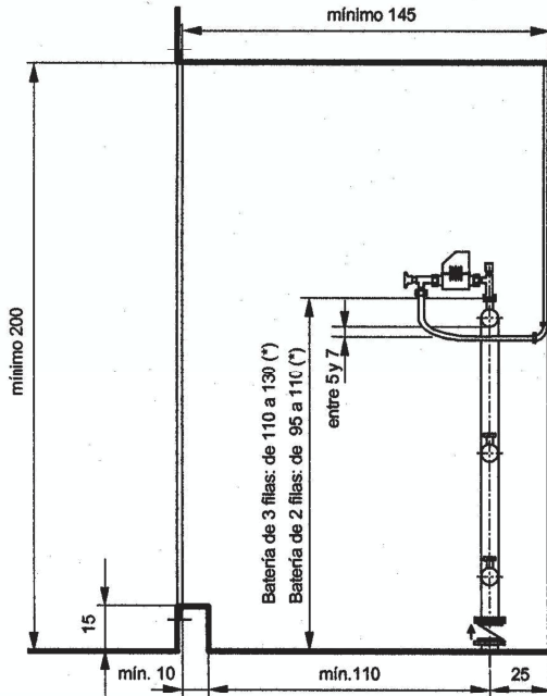
CUARTO BATERÍA SECCIÓN TRANSVERSAL
