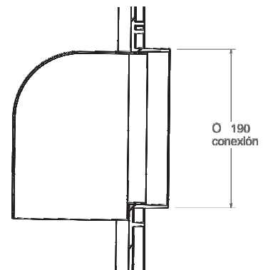
DETALLE B
