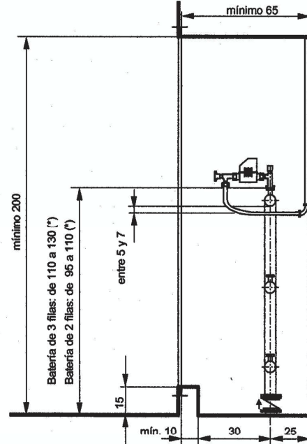
ARMARIO BATERÍA PLANTA
